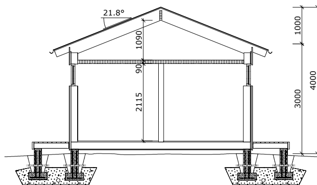
SEKTION A-A 1:100
