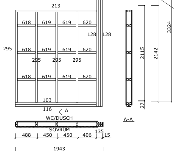
BÄRANDE INNERVÄGG IV-6 1:50
