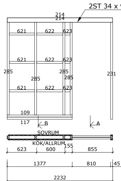
INNERVÄGG IV-5 1:50
