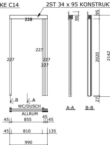
INNERVÄGG IV-7 1:50
