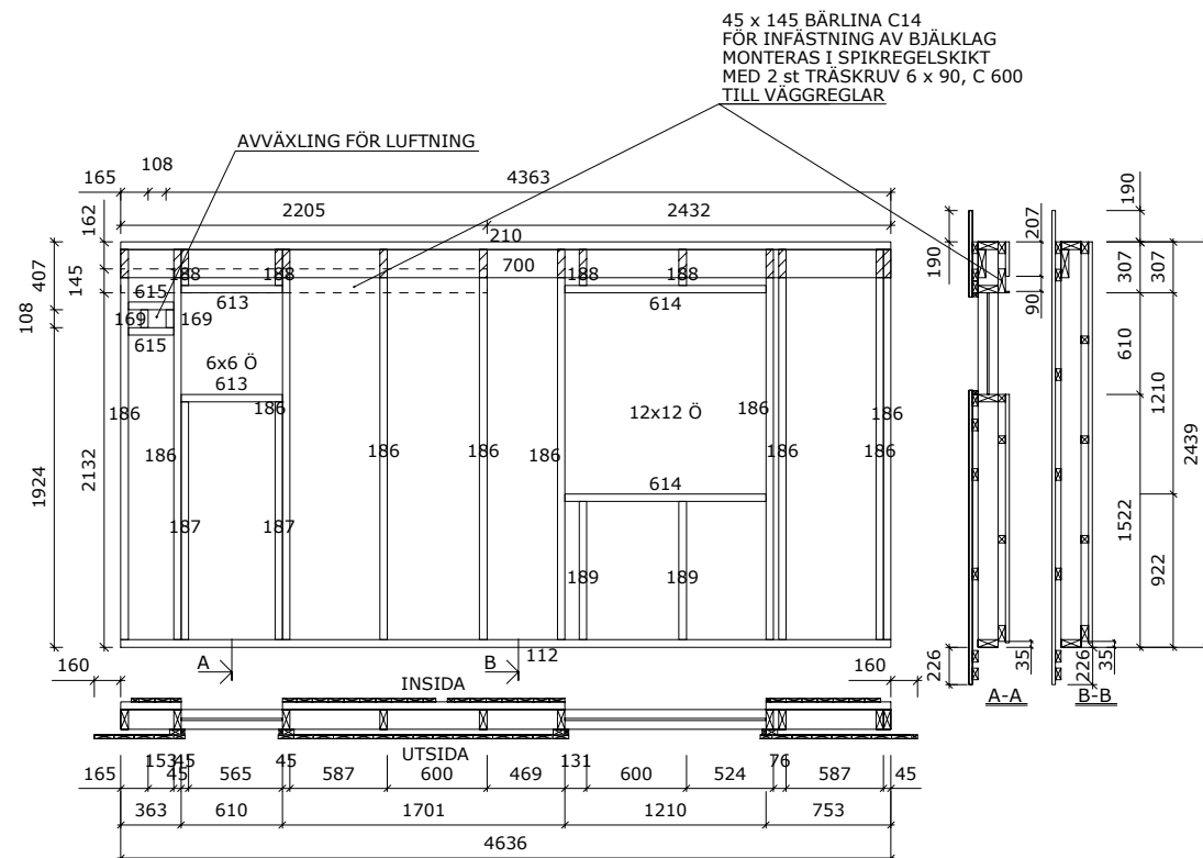
Yttervägg YV-4 1:50
