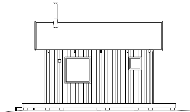
FASAD 2, 1:100
