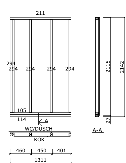
INNERVÄGG IV-9 1:50
