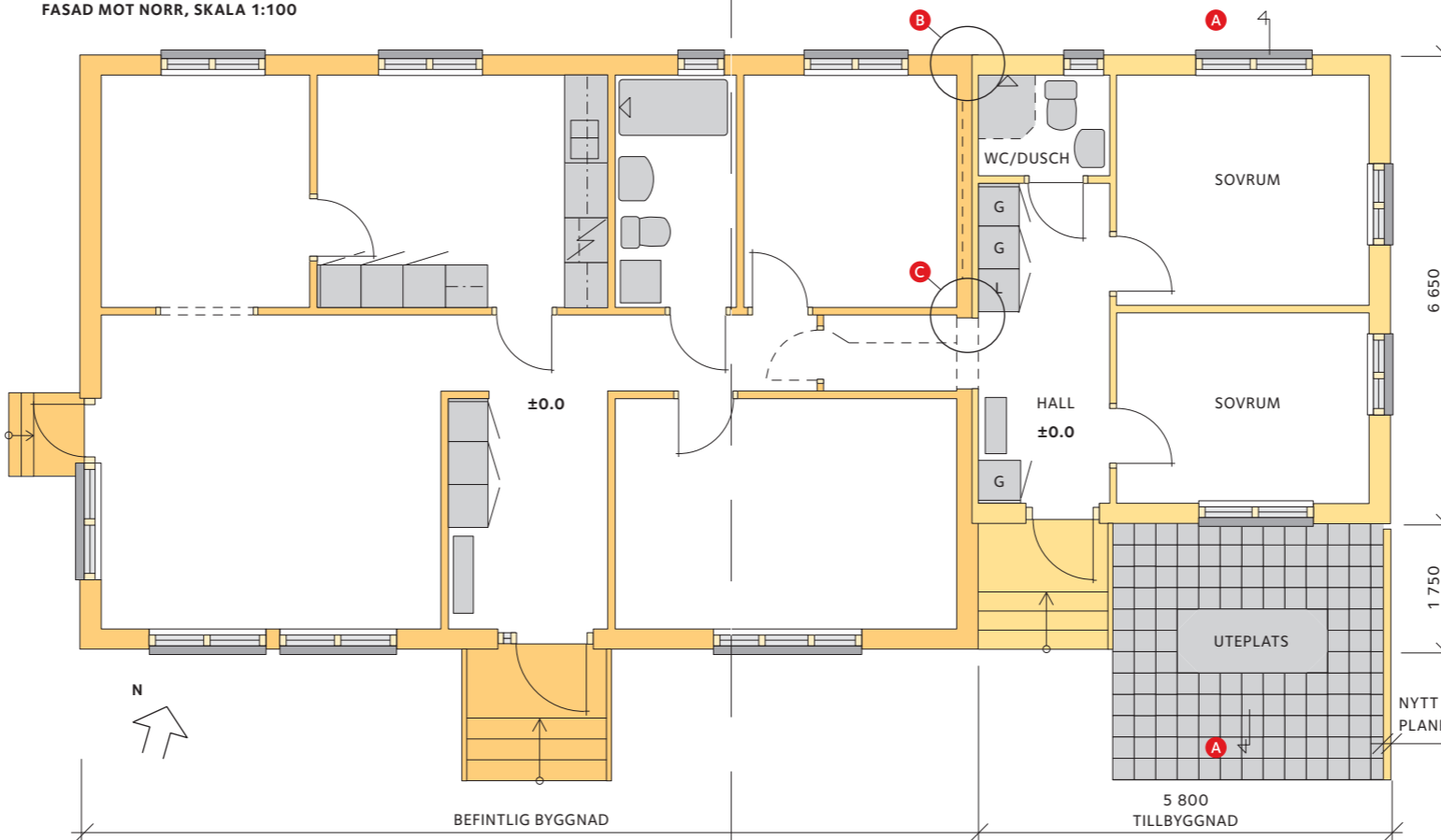
PLAN, SKALA 1:100
