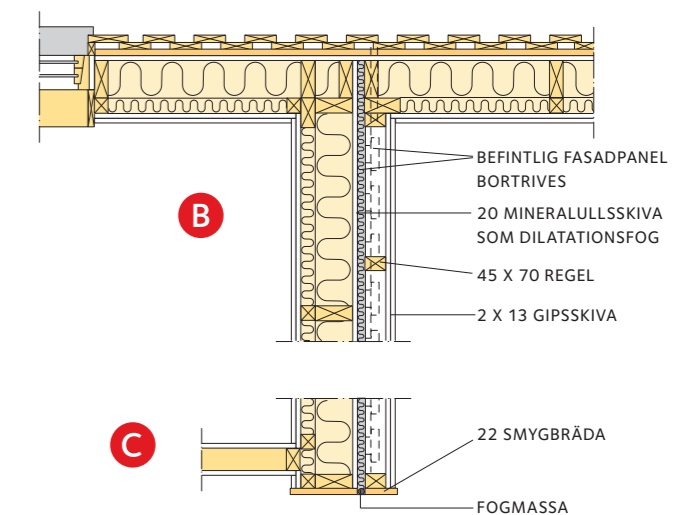
TILLBYGGNADENS ANSLUTNING MED DEN BEFINTLIGA BYGGNADEN
