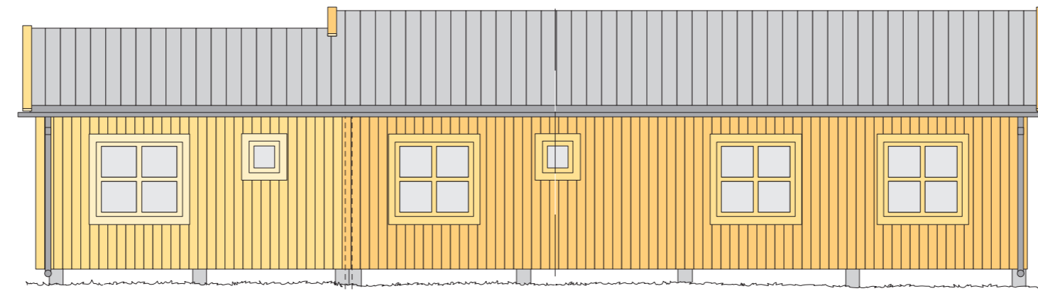
FASAD MOT SÖDER, SKALA 1:100
