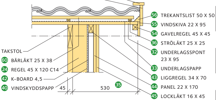
VERTIKALSNITT AV GAVELSPRÅNG
